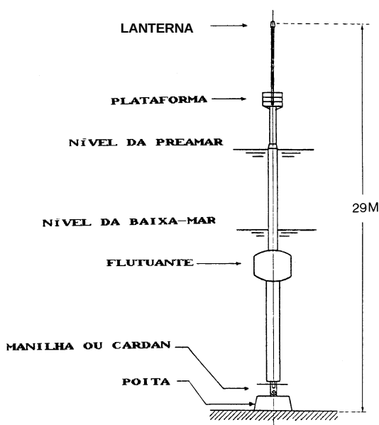
Figura 13.12 - Baliza articulada
