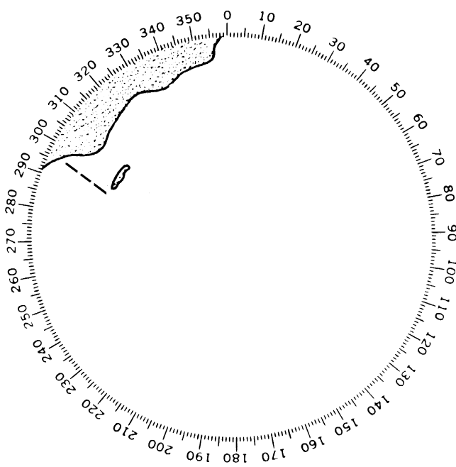
Figura 14.33 - Sinal codificado de RACON ("0")
