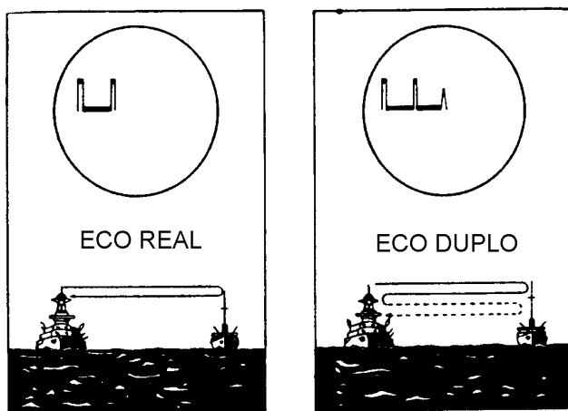
Figura 14.22 - Formação de Eco Múltiplo
