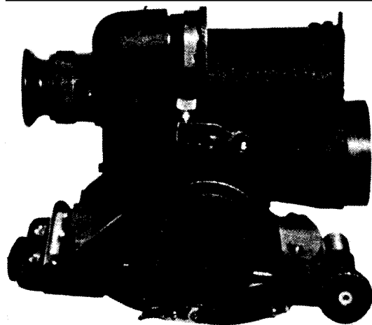
Figura 11.7 - Alidade Auto-Síncrona
