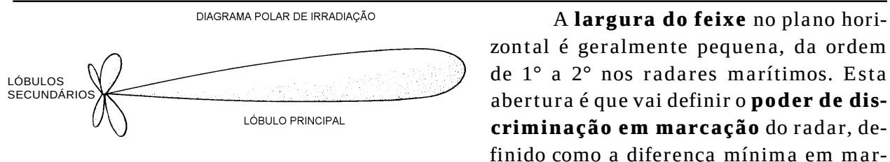
Figura 14.2 - Diagrama Polar Horizontal de Irradiação
