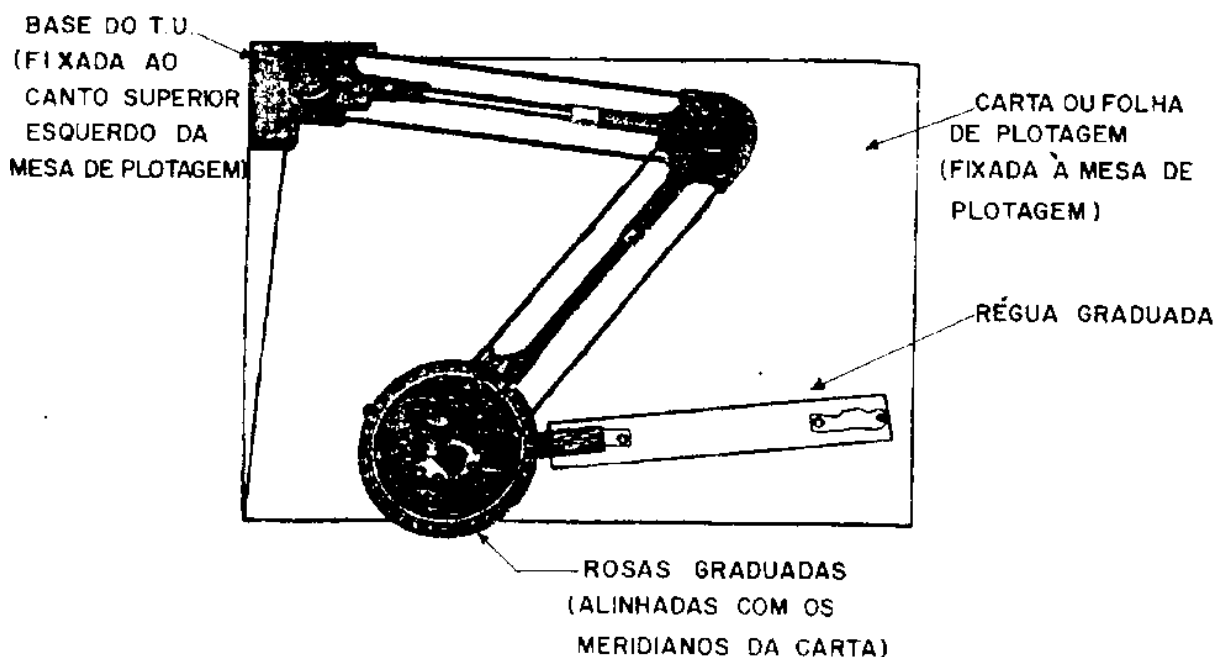
Figura 5.15 – Transferidor universal
