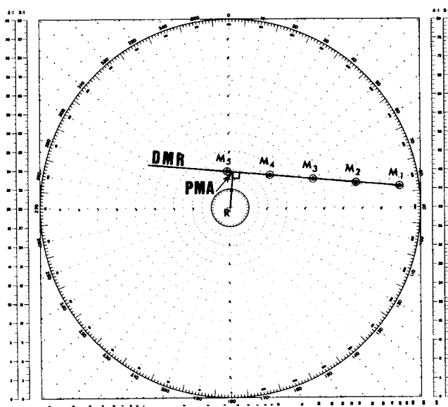
Figura 14.61 - Plotagem relativa na rosa de manobra
