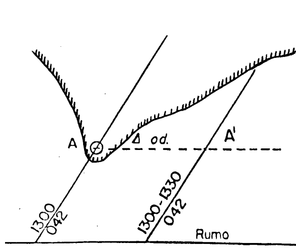
Figura 6.1 – Transporte de LDP – Reta de Marcação
