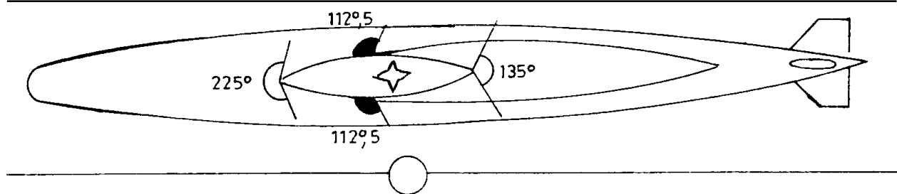
Figura 15.34 (a) - Submarino navegando na superfície, exibindo, além das luzes previstas no RIPEAM, luz âmbar intermitente
