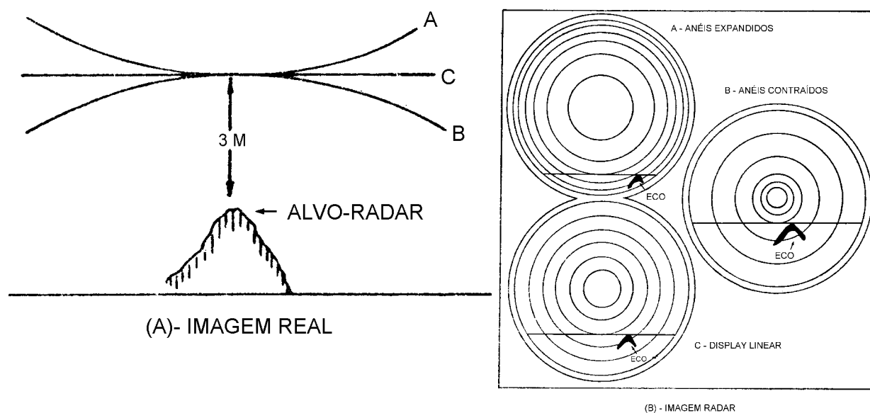
Figura 14.48 - Linearidade
