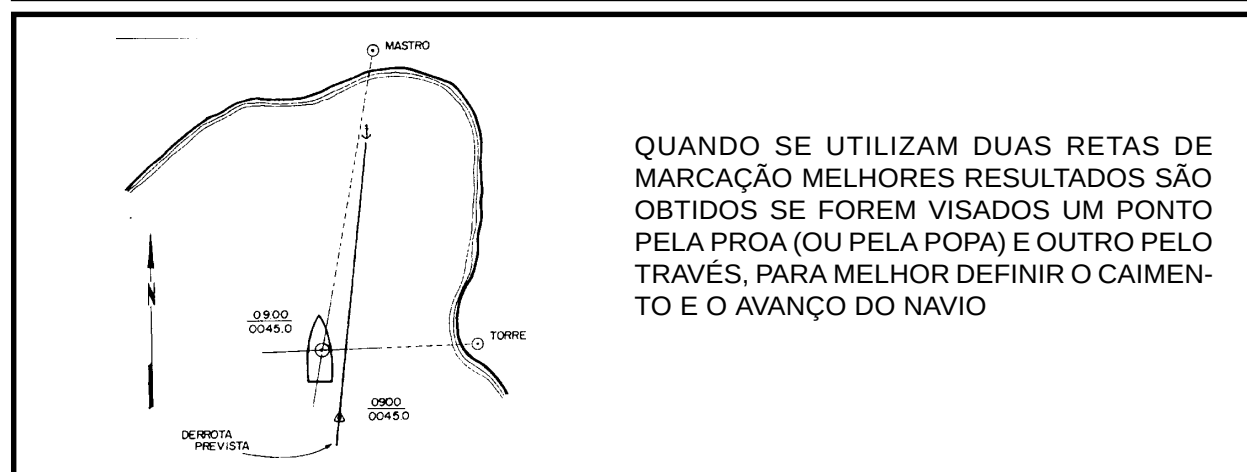
Figura 4.37 - Posição por interseção de duas retas de marcação – definição de caimento e avanço (ou atraso)
