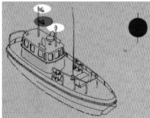
Figura 15.33 - Embarcação de praticagem, menor que 50 metros, fundeada
