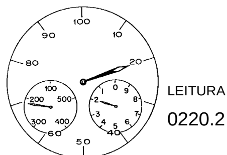
Figura 11.13 - Leitura do registrador
